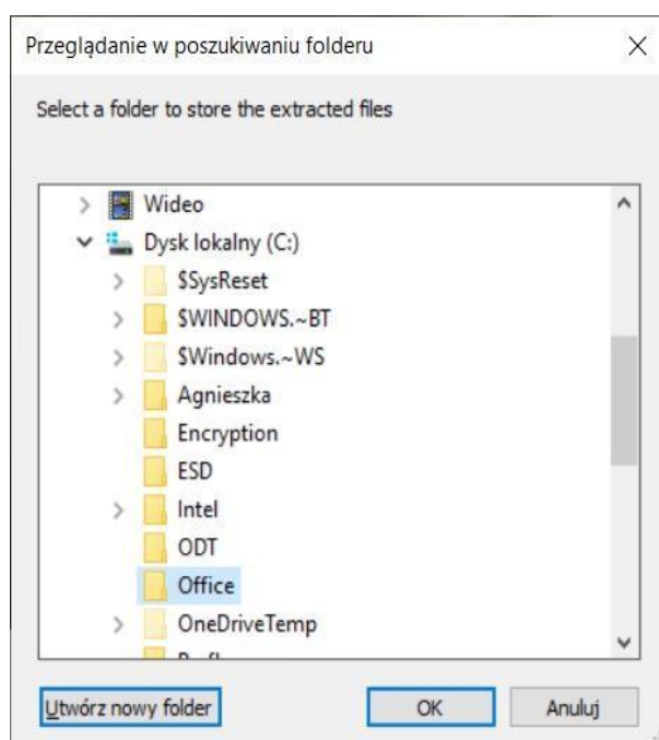
Rys. 1 Wypakowanie folderu
