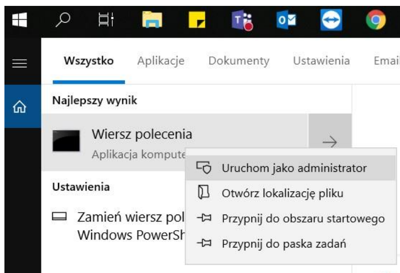
Rys. 3 Wiersz poleceń
